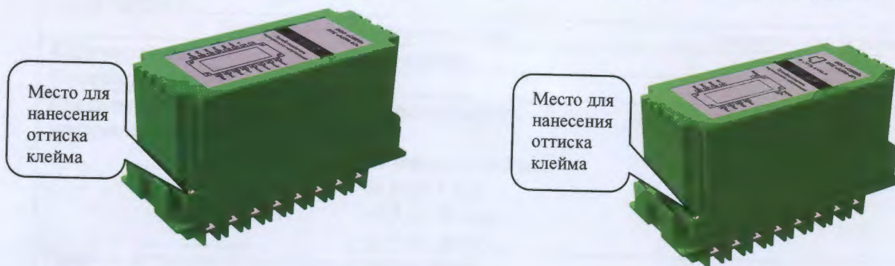
Рисунок 3 - Внешний вид измерительных преобразователей
